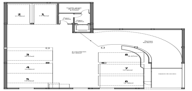
PLANTA SEMISÓTANO GENERAL
