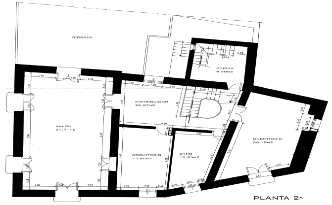
PLANTA 2ª
